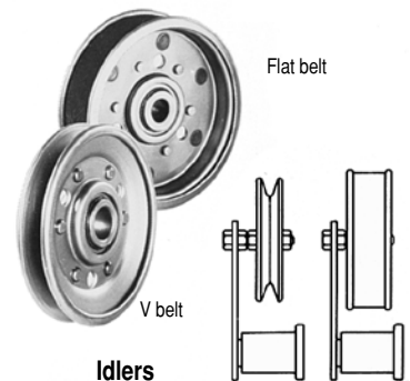
Idlers
