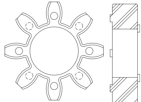
Standarddesign des Kupplungssterns
