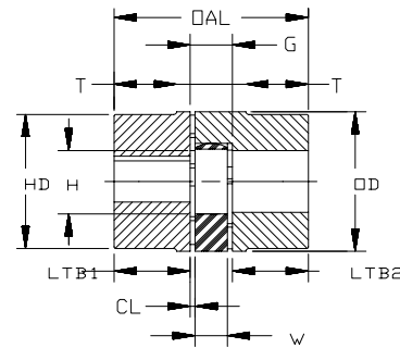
Ausführung 2 - Zwei „B“-Naben
